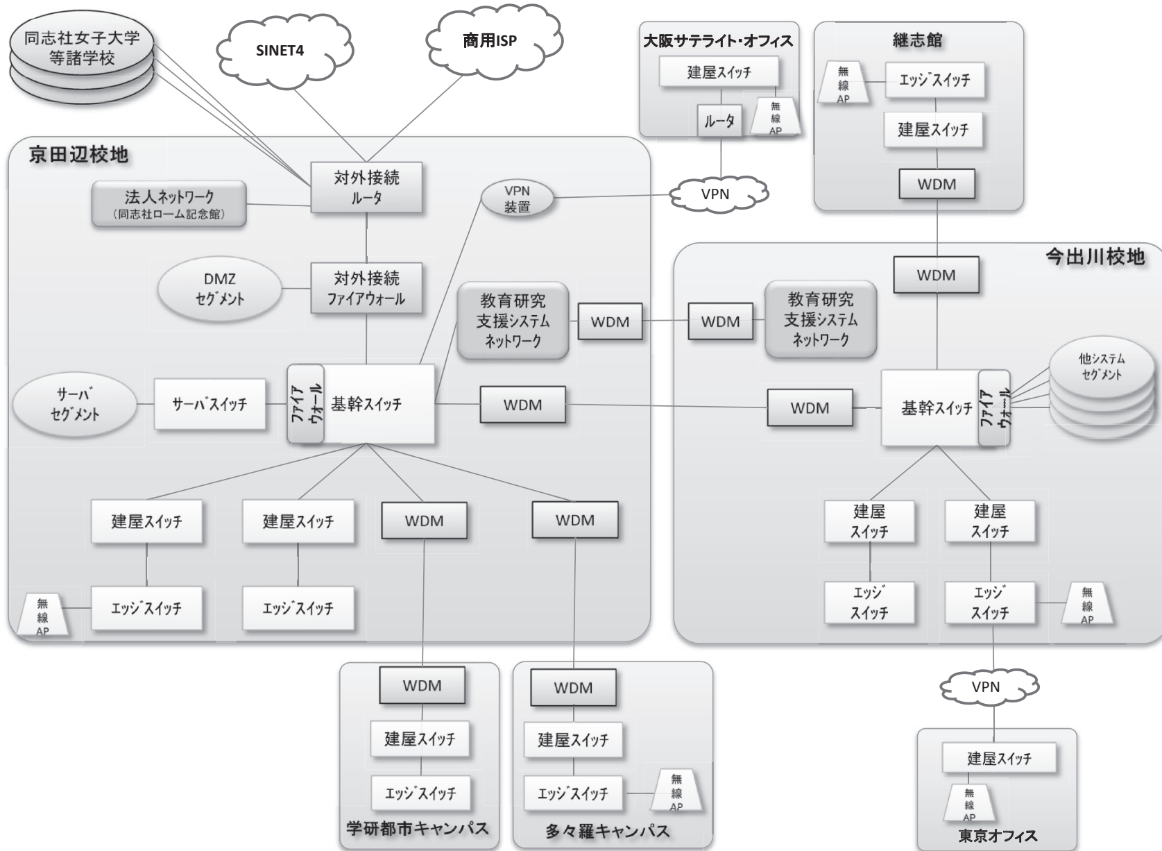
同志社大学 全学ネットワーク構成概略図
